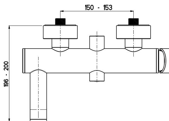
FAUCET BATH
